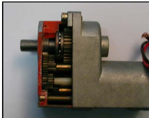
.Motoriduttore sezionato
